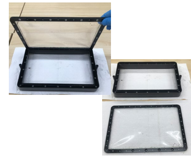
③ フレームごとフィルムを取り外します。
