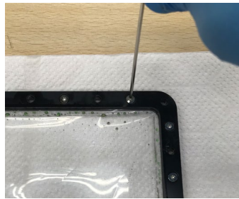
④ 取り出したフレームを裏返し、見えているネジをすべて取り外します。
