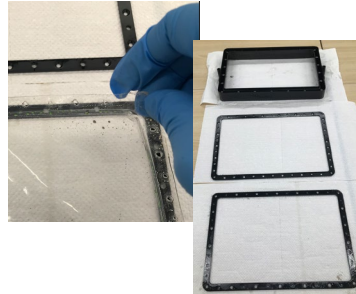
⑤ フレームを取り外し、レジンバット本体と共にあらためて清掃します。
